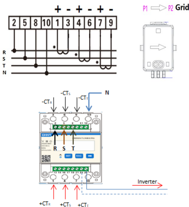
Figura 161 - Collegamenti Meter e sensori
