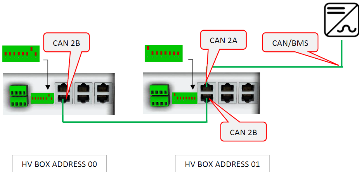
Figura 103 - Connessioni comunicazione fra le Torri batterie
