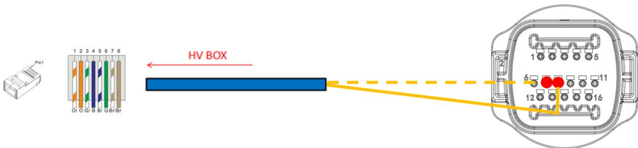
Figura 110 - Schema connessioni COM
