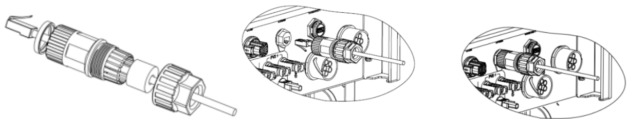
Figura 151 - Collegamento interfaccia DRMs (2)
