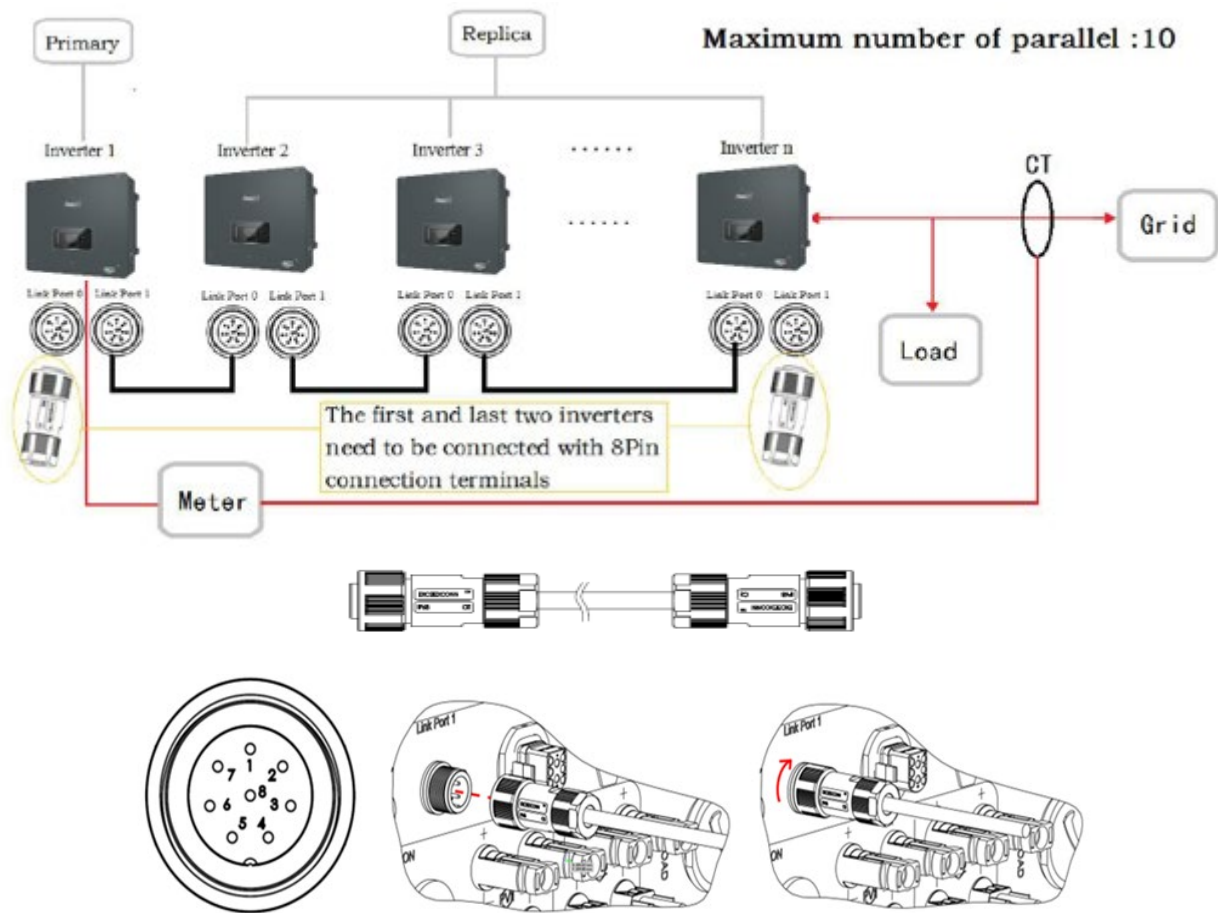
Figura 171 - Connessioni di parallelo fra inverter
