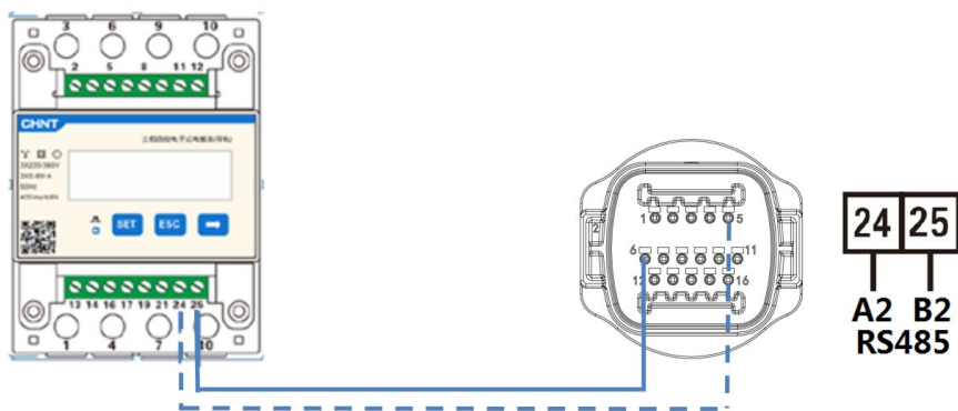
Figura 165 - Collegamento porta seriale Meter "a incastro"
