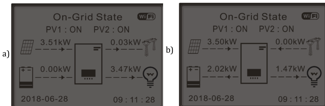
Figura 174 - Display inverter in modalità automatica
