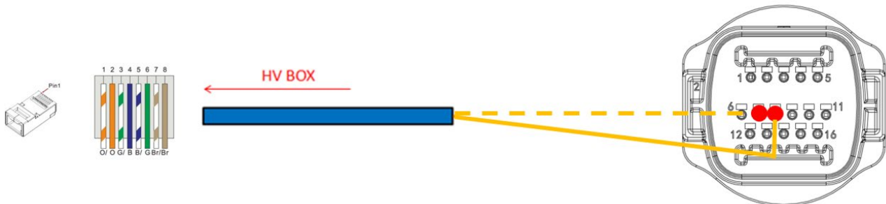
Figura 86 - Schema connessioni COM "a incastro"
