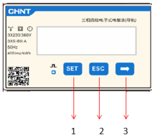
Figura 169 - Legenda Meter
