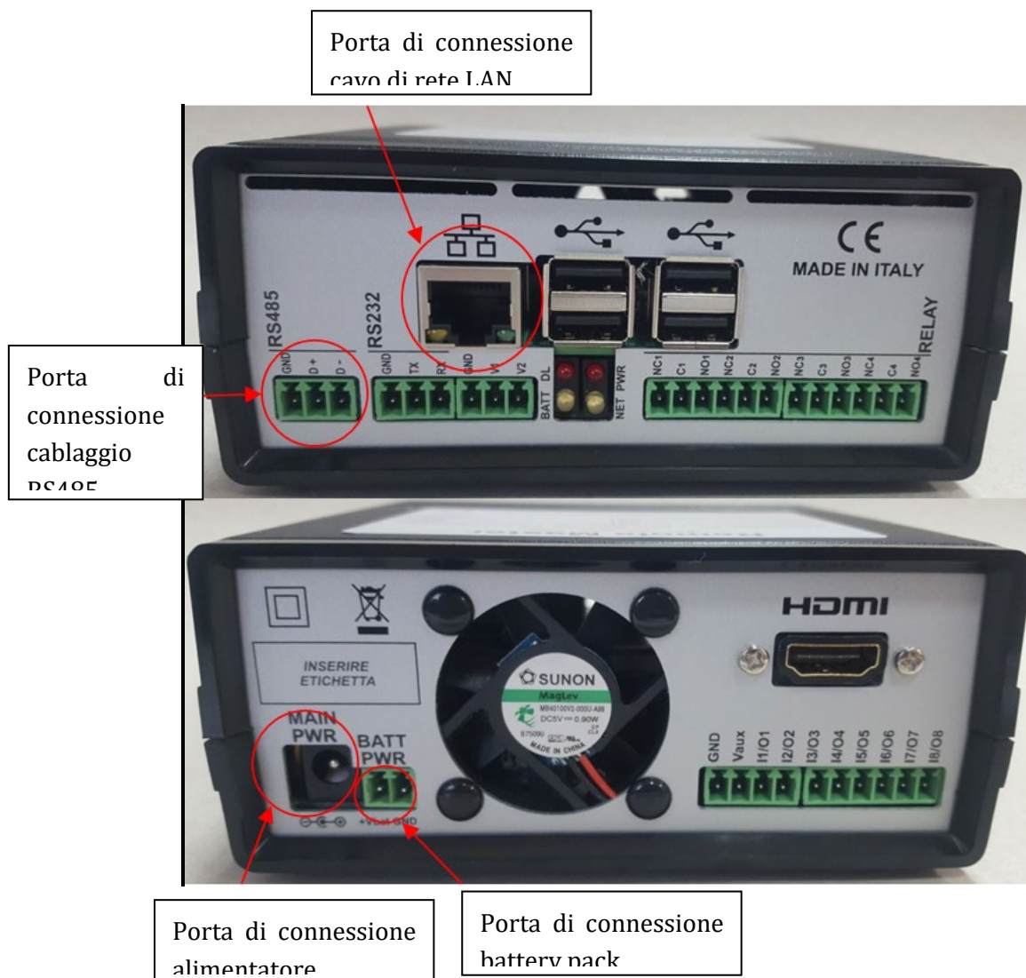
Figura 244: Back Datalogger
