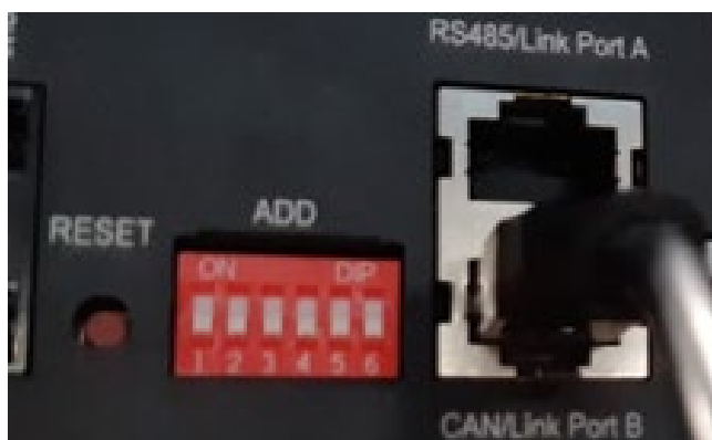
Figura 33 - Address batteria 000000
