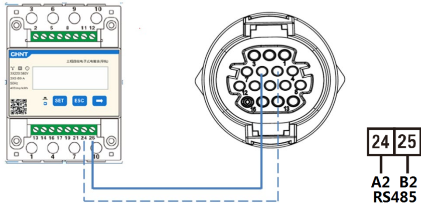
Figura 164 - Collegamento porta seriale Meter "a vite"
