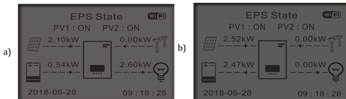
Figura 178 - Display con EPS in funzione
