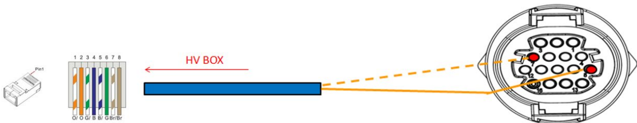
Figura 85 - Descrizione interfaccia COM "a vite"
