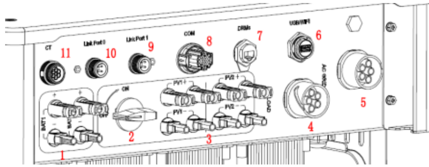
Figura 71 - Sezione connessioni Inverter
