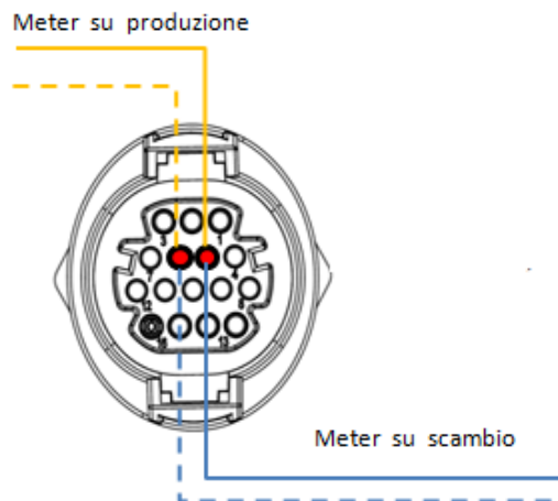
Figura 167 - Collegamento porta seriale COM "a vite" con più di un Meter
