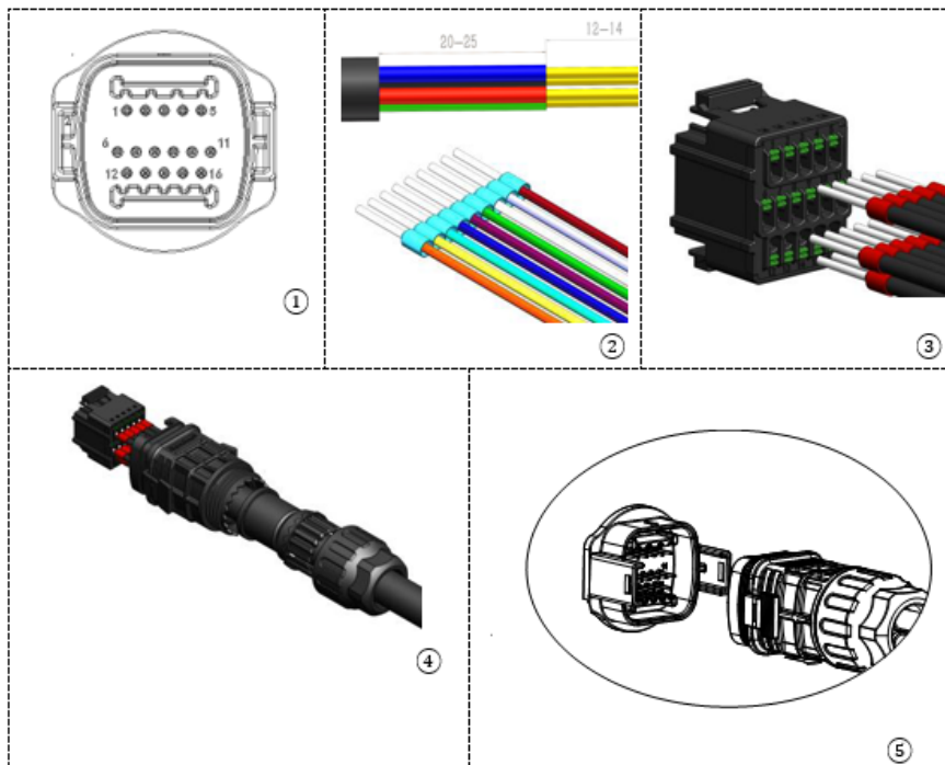
Figura 73 - Connessione porta COM "a incastro"
