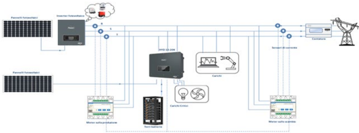
Figura 166 - Schema installazione Ibrido con Meter su scambio e produzione
