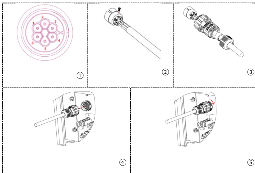
Figura 156 - Interfaccia CT
