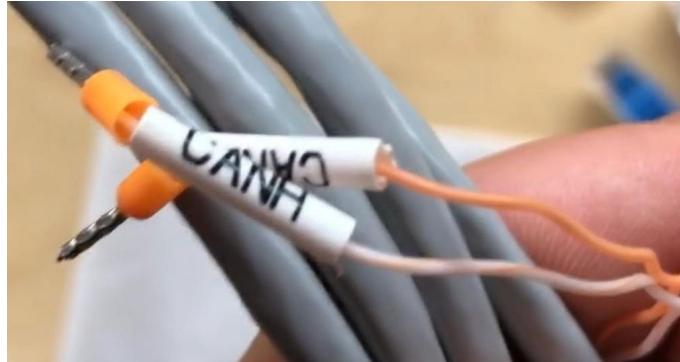
Figura 105 - Cavo comunicazione Inverter/HV BOX
