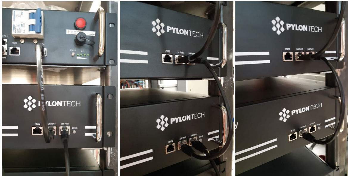
Figura 31 - Connessioni comunicazione: BMS e primo modulo batteria (sinistra), connessione fra moduli batteria (al centro), connessione fra penultimo ed ultimo modulo batteria della serie (destra)
