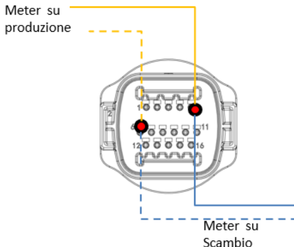
Figura 168 - Collegamento porta seriale COM “a incastro” con più di un Meter
