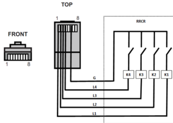
Figura 152 - Connessione RRCR
