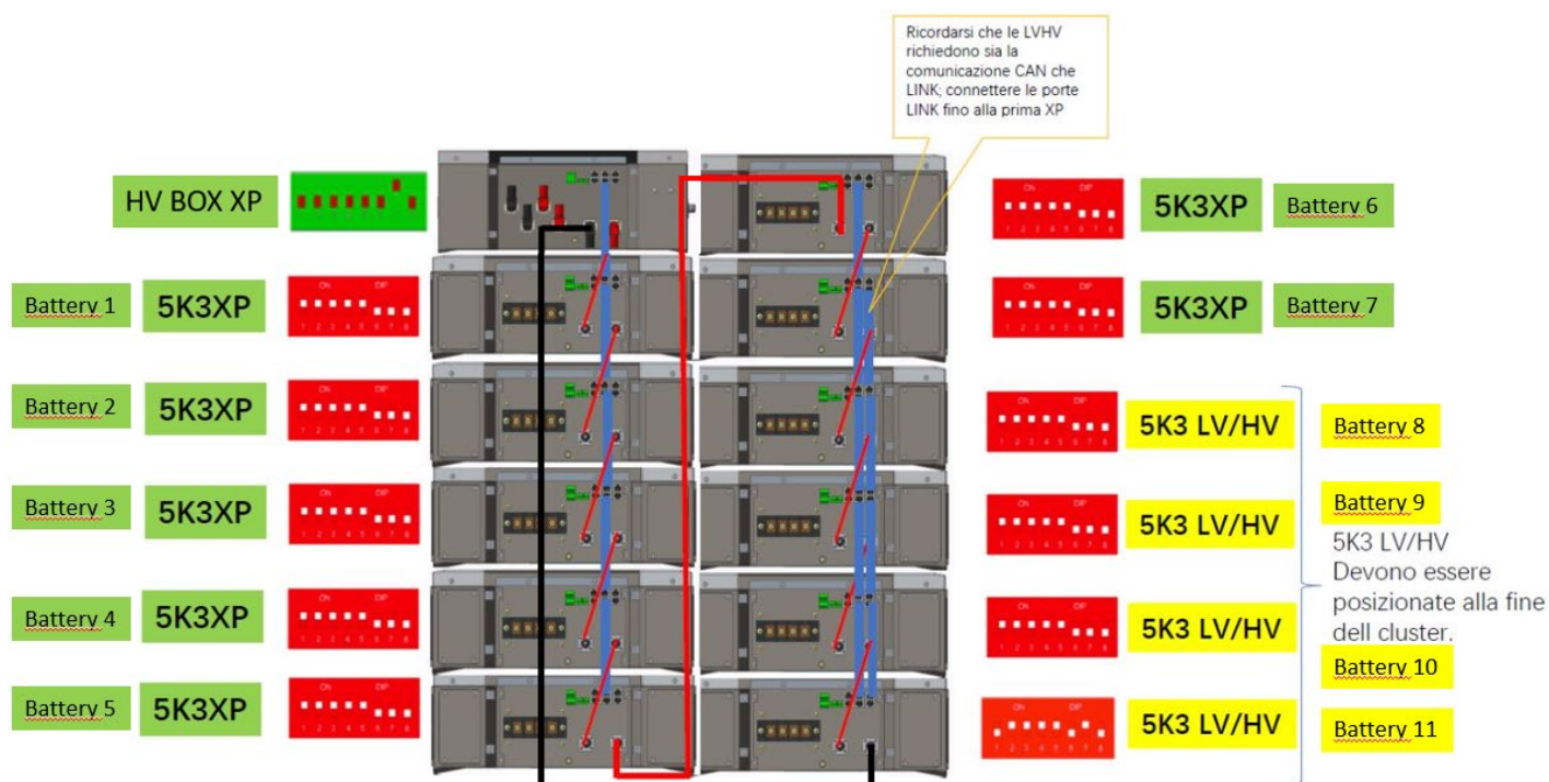
Figura 112 - Connessione potenza e comunicazione batterie 5K3 e 5K3XP
