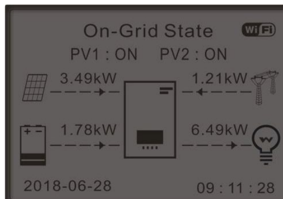
Figura 176 - Display inverter in modalità autoconsumo
