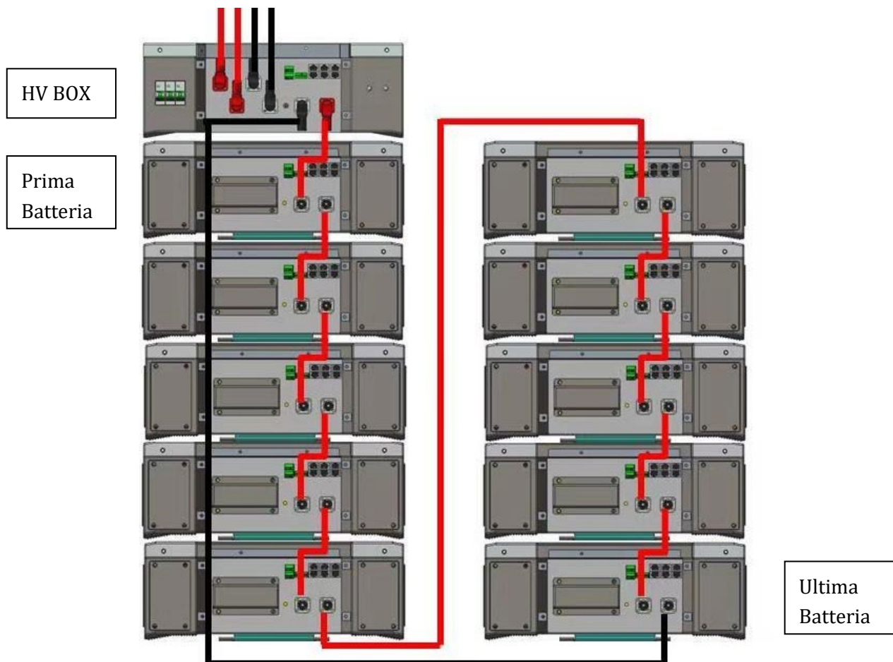
Figura 99 - Cablaggio potenza fra moduli batterie in serie
