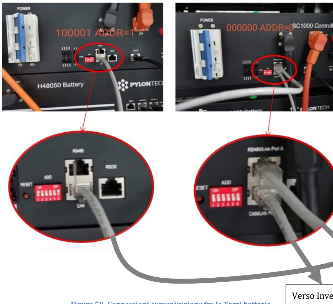
Figura 50- Connessioni comunicazione fra le Torri batterie
