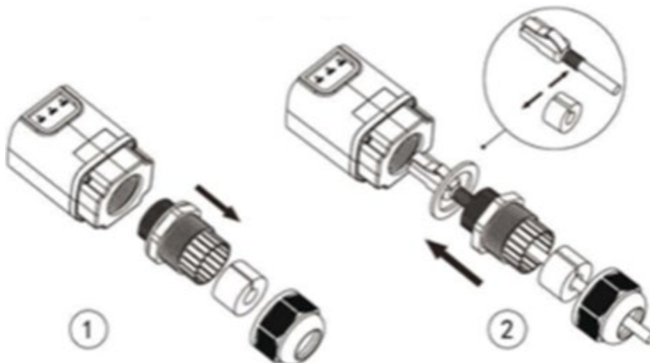
Figura 204 – Inserimento del cavo di rete all'interno del dispositivo
