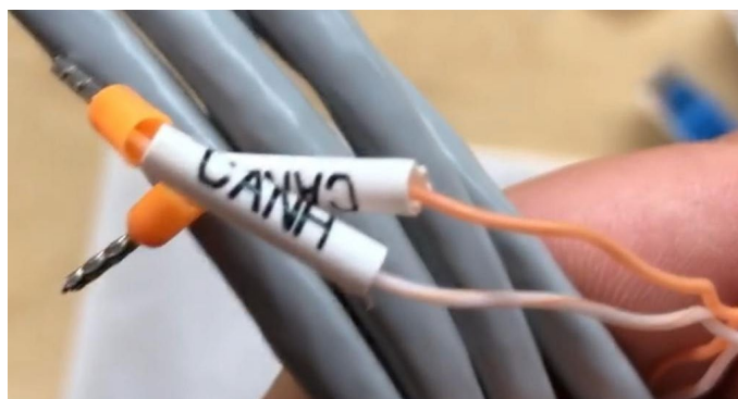
Figura 93 - Cavo comunicazione Inverter/HV BOX
