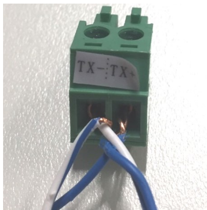
Figura 220 - Serraggio del cavo di rete sul morsetto RS485
