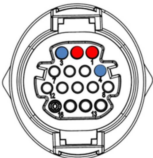
Figura 222 - Collegamento della linea seriale tramite connettore di comunicazione per 3PH HYD5000-HYD20000-ZSS
