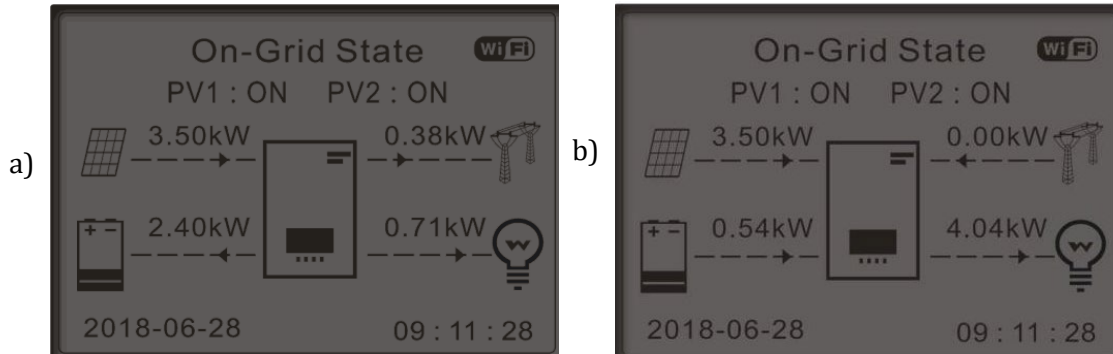
Figura 175 - Display inverter in modalità automatica
