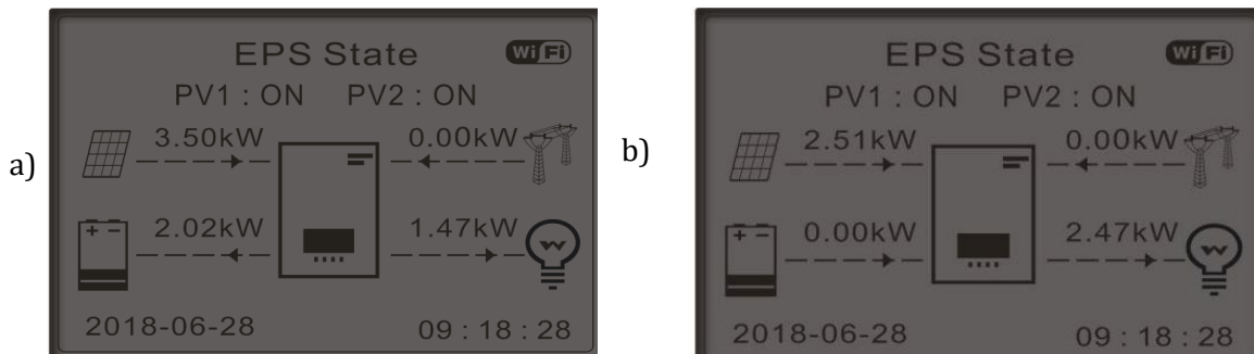
Figura 177 - Display con EPS in funzione
