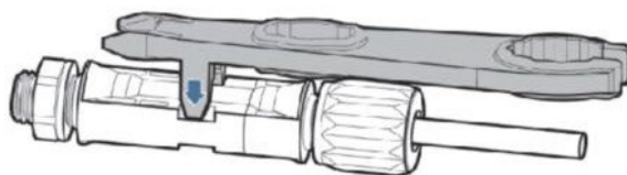
Figura 23 – Scollegamento dei connettori fotovoltaici
