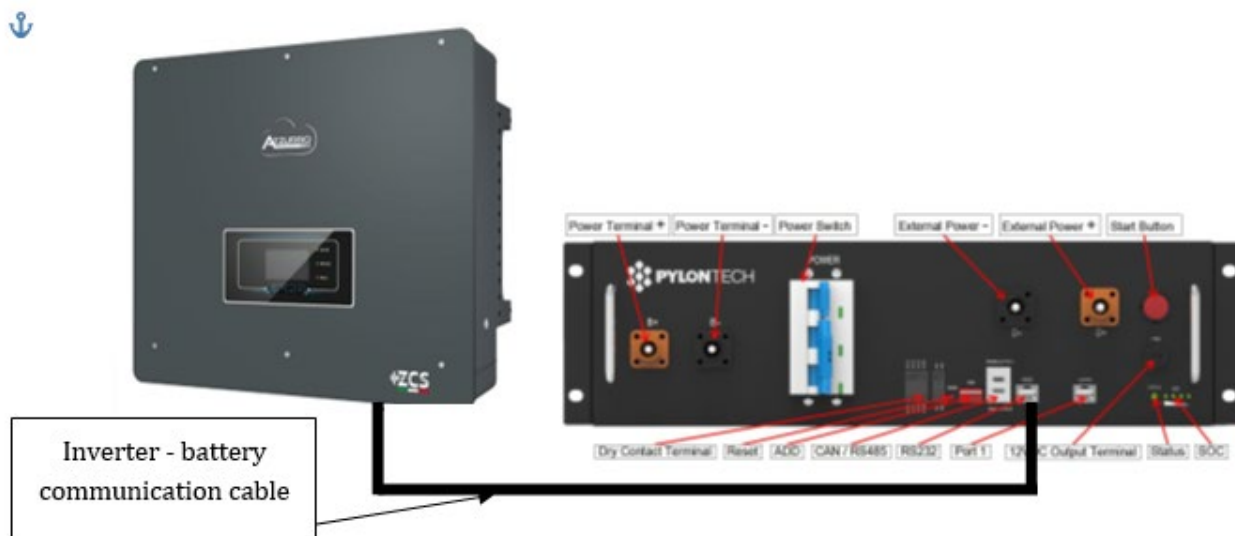
Figura 32 - Connessione comunicazione inverter ibrido e BMS
