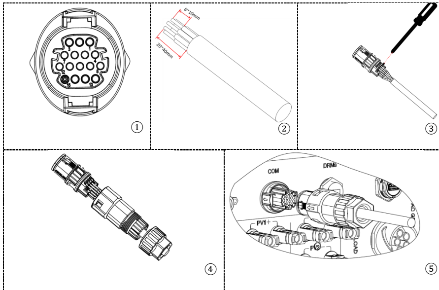
Figura 162 – Interfaccia COM “a vite”
