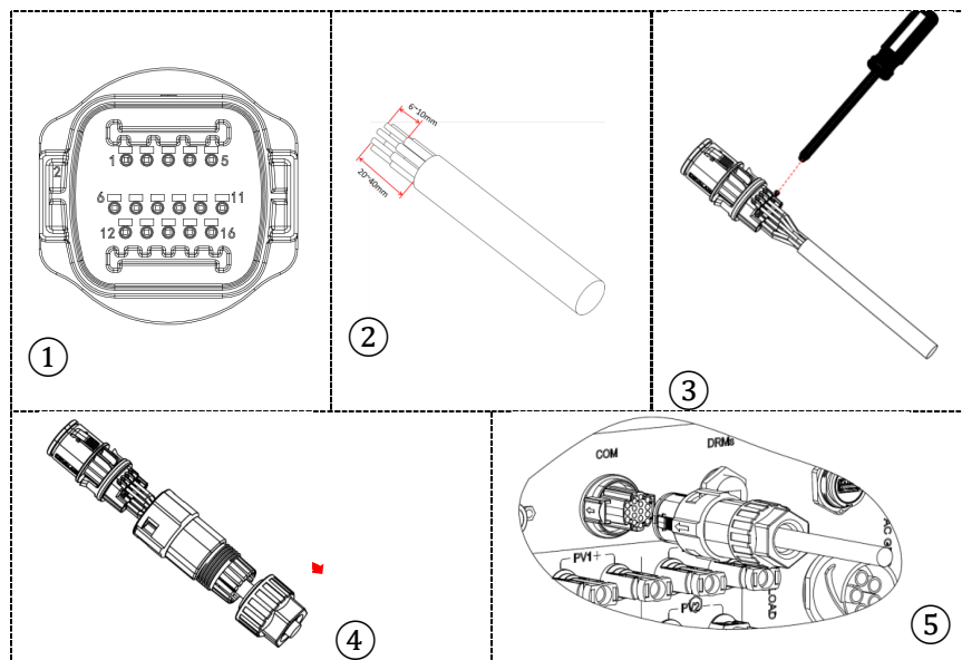
Figura 96 - Connessione porta COM "a incastro"
