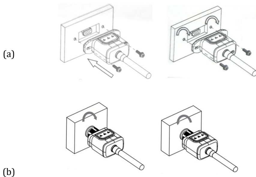
Figura 180 - Inserimento e fissaggio della scheda wifi esterna
