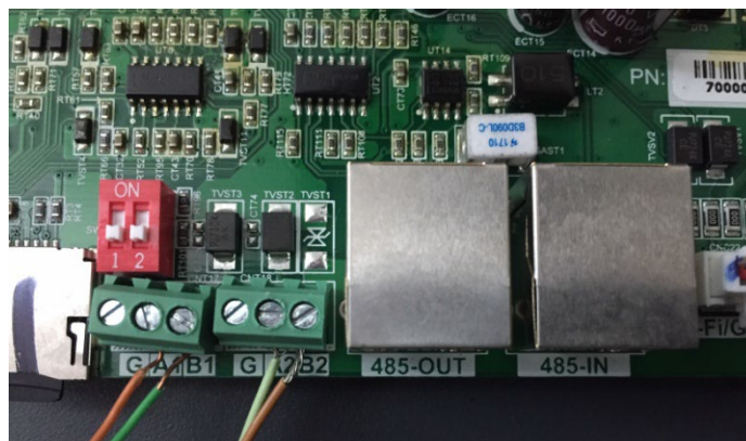
Figura 221 - Collegamento linea seriale tramite morsettiera RS485 e tramite plug RJ45
