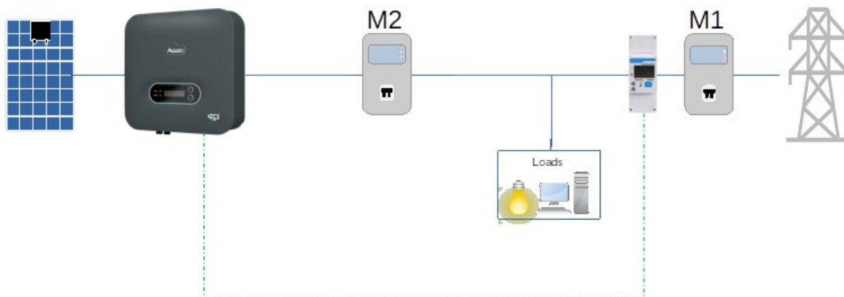
Figura 1 - posizione logica del meter DDSU666
