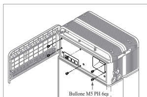
Bullone M5 PH 6ca
