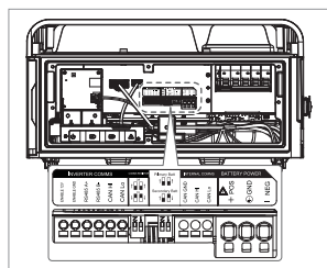
Foro #2 Cavo di comunicazione
