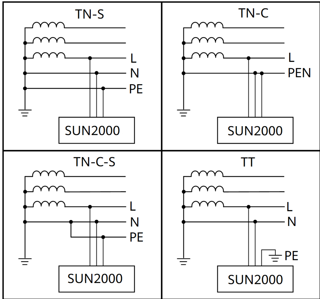
Figura 2-4 Tipi di rete elettrica
