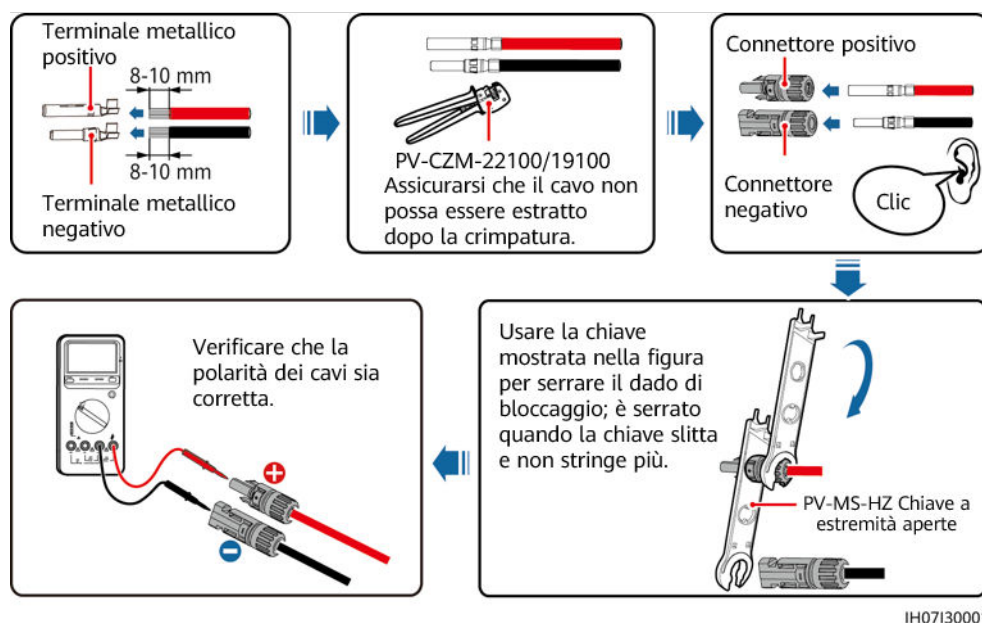
Figura 5-14 Assemblaggio di un connettore CC
