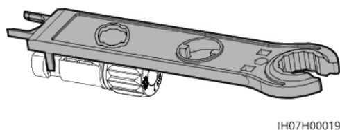
Figura 5-16 Rimozione di un connettore CC
