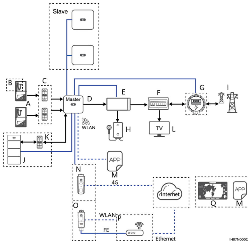
Figura 2-3 Scenario SUN2000 in cascata (i riquadri tratteggiati indicano le configurazioni facoltative)
