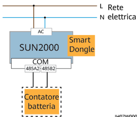
Figura 5-19 SUN2000 singolo
