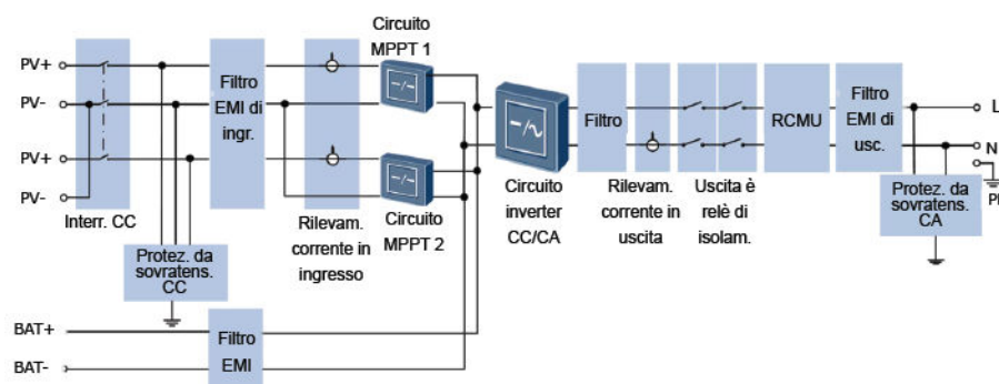
Figura 2-7 Diagramma schematico
