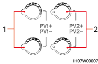
Figura 5-13 Terminali di ingresso CC
